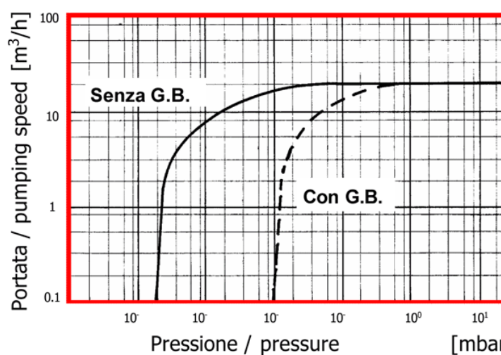
Curve di portata – Pumping speed
